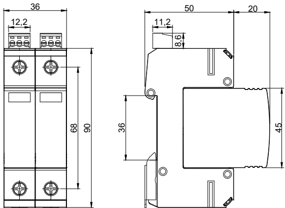
Габаритные размеры
