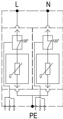
Принципиальная схема
